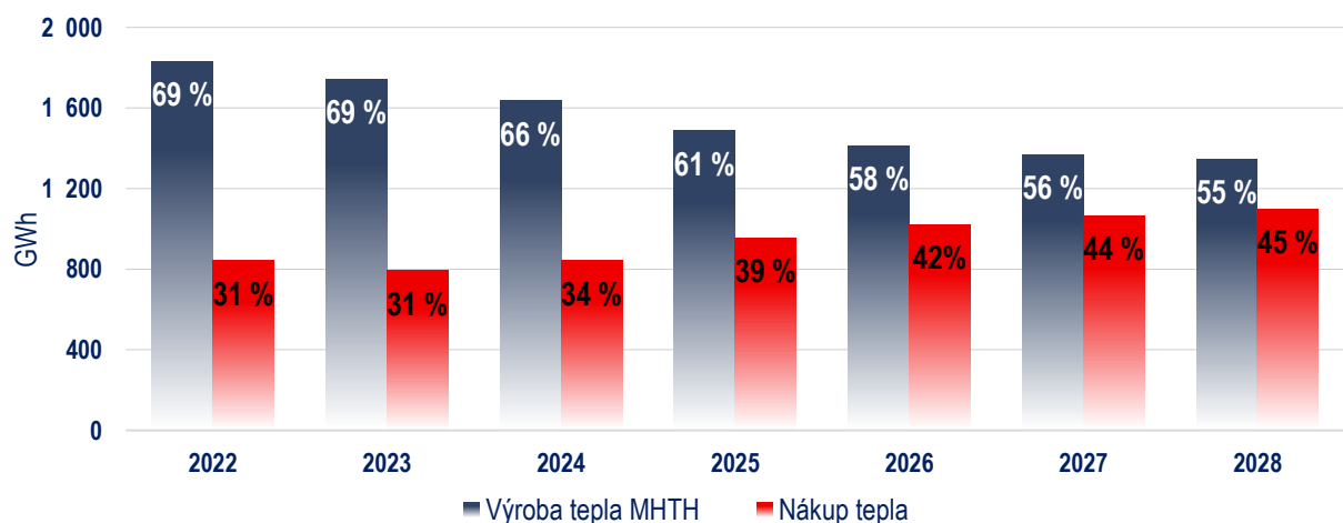
Graf 8: Podiel nakupovaného tepla
