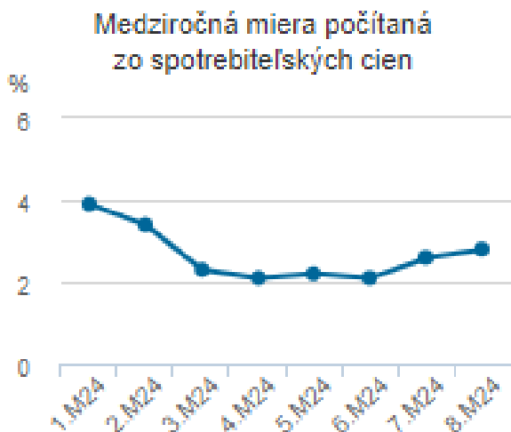
Graf 9: Inflácia
